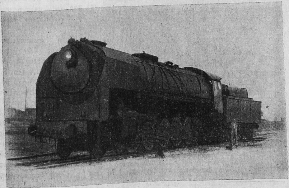
Ἡ νέα ἰσχυρωτάτη ἀτμάμαξα τῶν ΣΕΚ, σειρᾶς Μα
